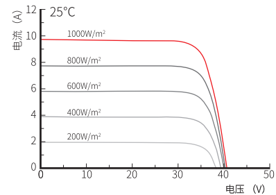
电流-电压曲线 (LR6-60HBD 310W)
