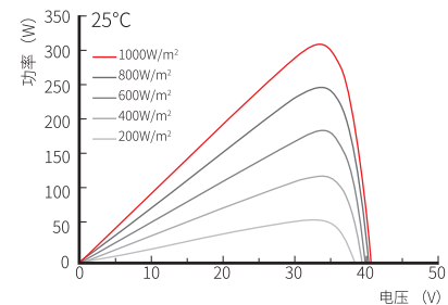
功率-电压曲线 (LR6-60HBD 310W)
